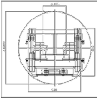
立坑設置図
