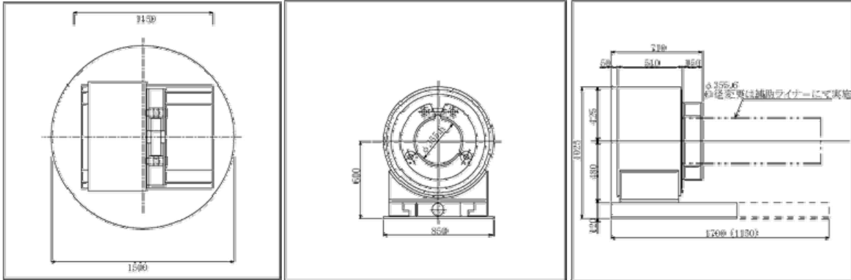
立坑設置図
