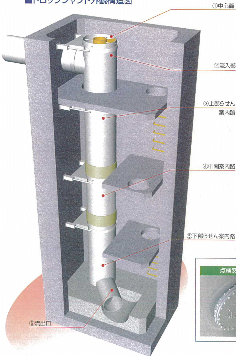
■ドロップシャフト外観構造図
